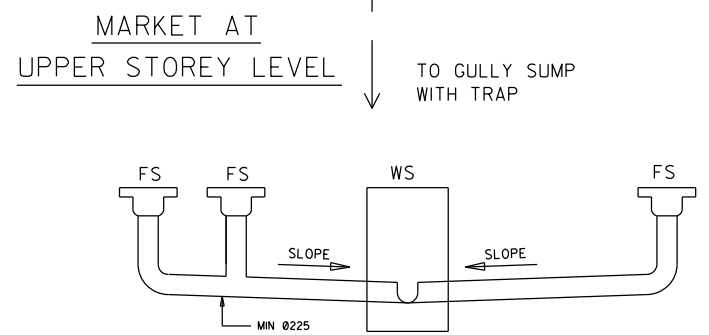
ELEVATION A - A
