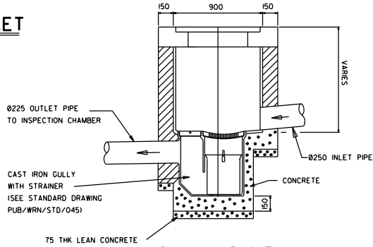
GULLY SUMP
